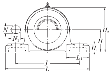
Тип со стальной штампованной пылезащитной крышкой Сквозная Z-UCP...D1 Несквозная ZM-UCP...D1
