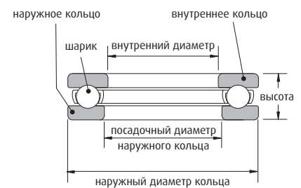
Однорядный упорный шарикоподшипник
