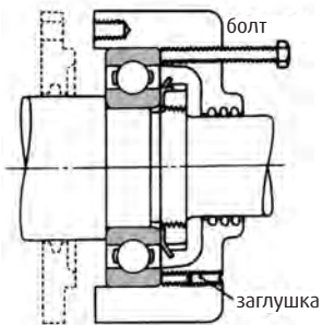
Извлечение наружного кольца при помощи демонирующих болтов
