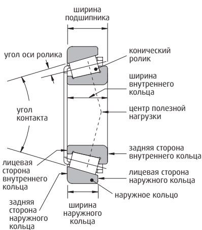
Конический роликоподшипник
