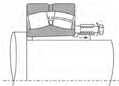
Удаление стяжной втулки при помощи отжимной гайки
