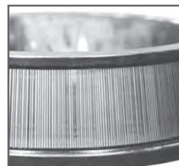
Электрическая коррозия
