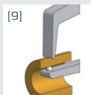
Резец R 0,4 мм Шарик Ø 1,5 мм
