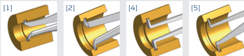
[1] Резец R 0,1 мм [2] Шарик Ø 0,6 мм Шарик Ø 1,0 мм Шарик Ø 1,3 мм [3] Шарик Ø 1,0 мм Шарик Ø 1,5 мм Шарик Ø 2,0 мм
