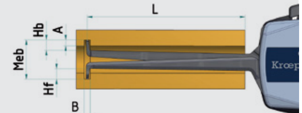
Meb Область измерения Hb Длина подвижного измер. контакта A Глубина паза Hf Длина жесткого измер. контакта B Глубина паза L Глубина измерения
