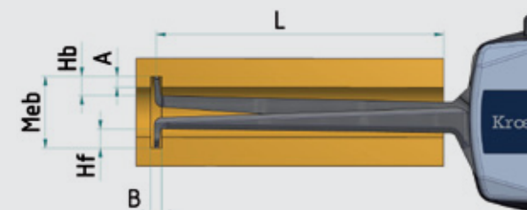
Meb Область измерения Hb Длина подвижного измер. контакта A Глубина паза Hf Длина жесткого измер. контакта B Глубина паза L Глубина измерения
