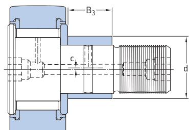
KRE .. PPA
