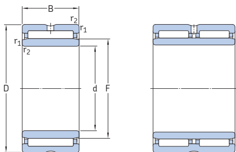
NKI(S) NA 49
