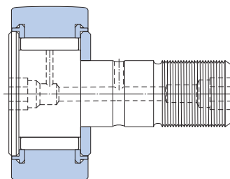
KRV .. PPA
