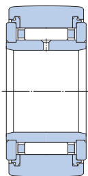
NATR .. PPA
