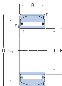
PNA
