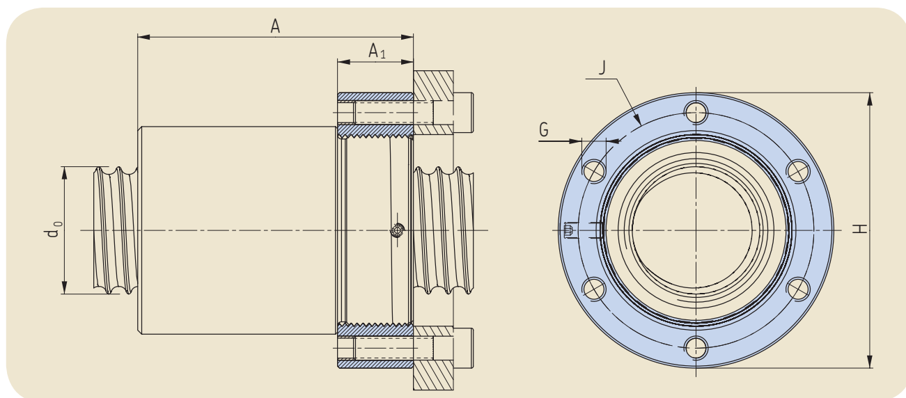
Flange
