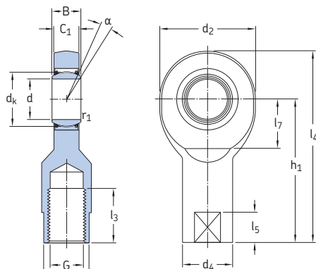
SI(L)..TXE-2LS
