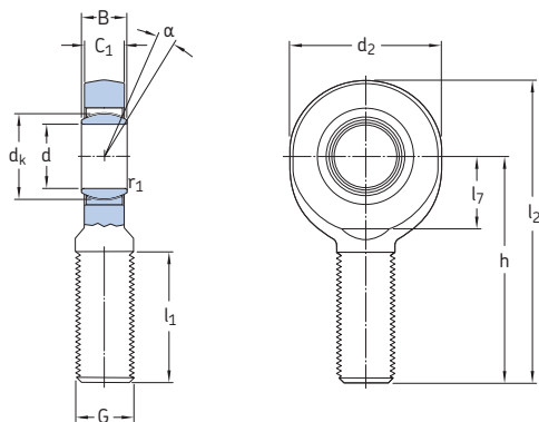
SA(L).. C
