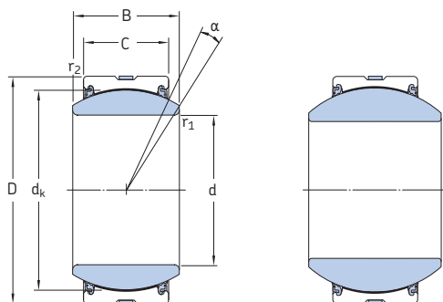
GE .. TX(G3)A-2LS
