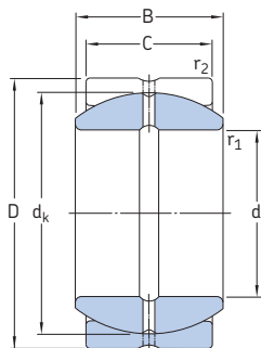
GEZ .. ES
