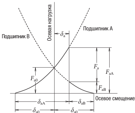
F_a : Осевая нагрузка, действующая извне F_{aA} : Осевая нагрузка на подшипник А F_{aB} : Осевая нагрузка на подшипник В \delta_a : Смещение дууплексных подшипников \delta_{aA} : Смещение подшипника А \delta_{aB} : Смещение подшипника В
