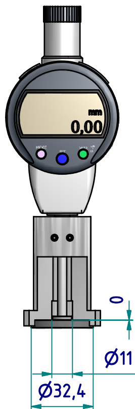
calibration ( 1 : 2 )
